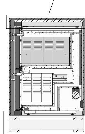
SEZIONE A-A
