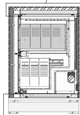
SEZIONE A-A
